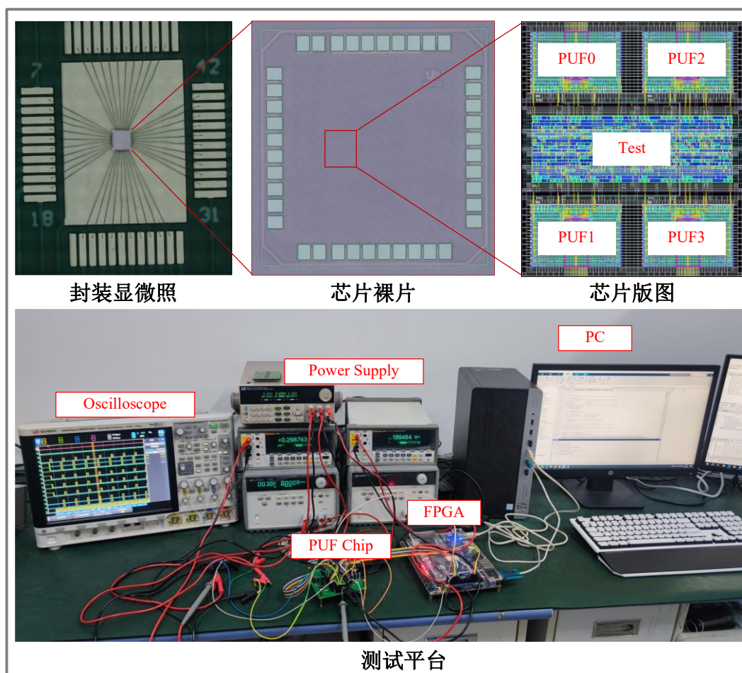
全定制 PUF 芯片与测试平台
